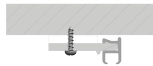
SYSTEM 200 Montage mit Deckenträger installation with ceiling bracket
